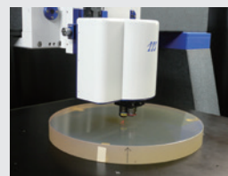
12吋玻璃基板平面度掃描
