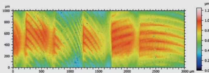
超精密加工模仁表面3D紋理掃描
