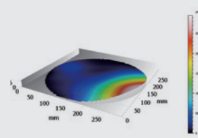
12吋玻璃基板平面度掃描
