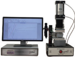
LT-451 介電固化監測儀
