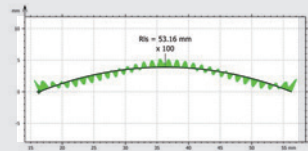
輪廓與表面微結構
