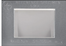
粗度標準片 Ra 0.02 ~ 6 µm
