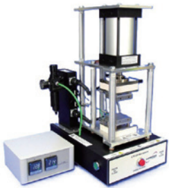
PCB 固化測試機 GFRP/CFRP 材料
