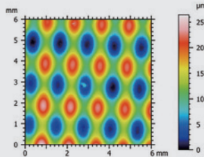
微結構 3D 掃描
