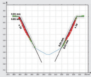
孔輪廓CAD擬合
